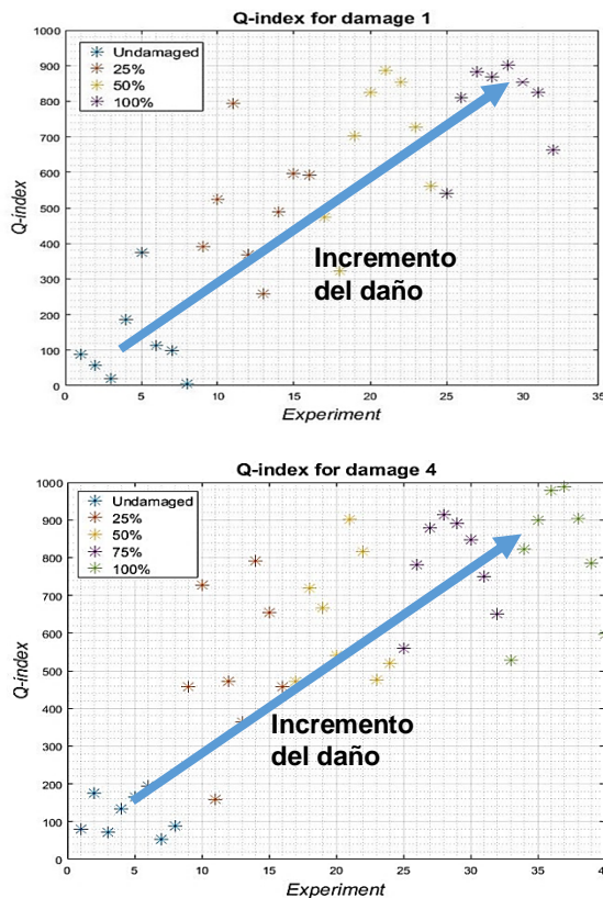
Figura 6. Resultados experimentales del índice Q para los casos de daño D1 (arriba) y D4 (abajo) en las condiciones sin daño, 25%, 50% y 100% de daño introducido.
